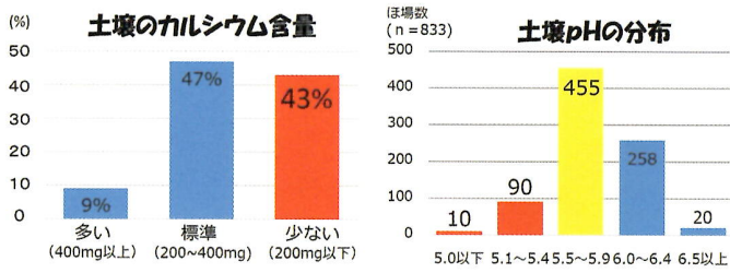
図1 根室管内A町の土壌pH(右)と土壌のカルシウム含量(左) (平成25~26年の土壌分析データ n=833)
